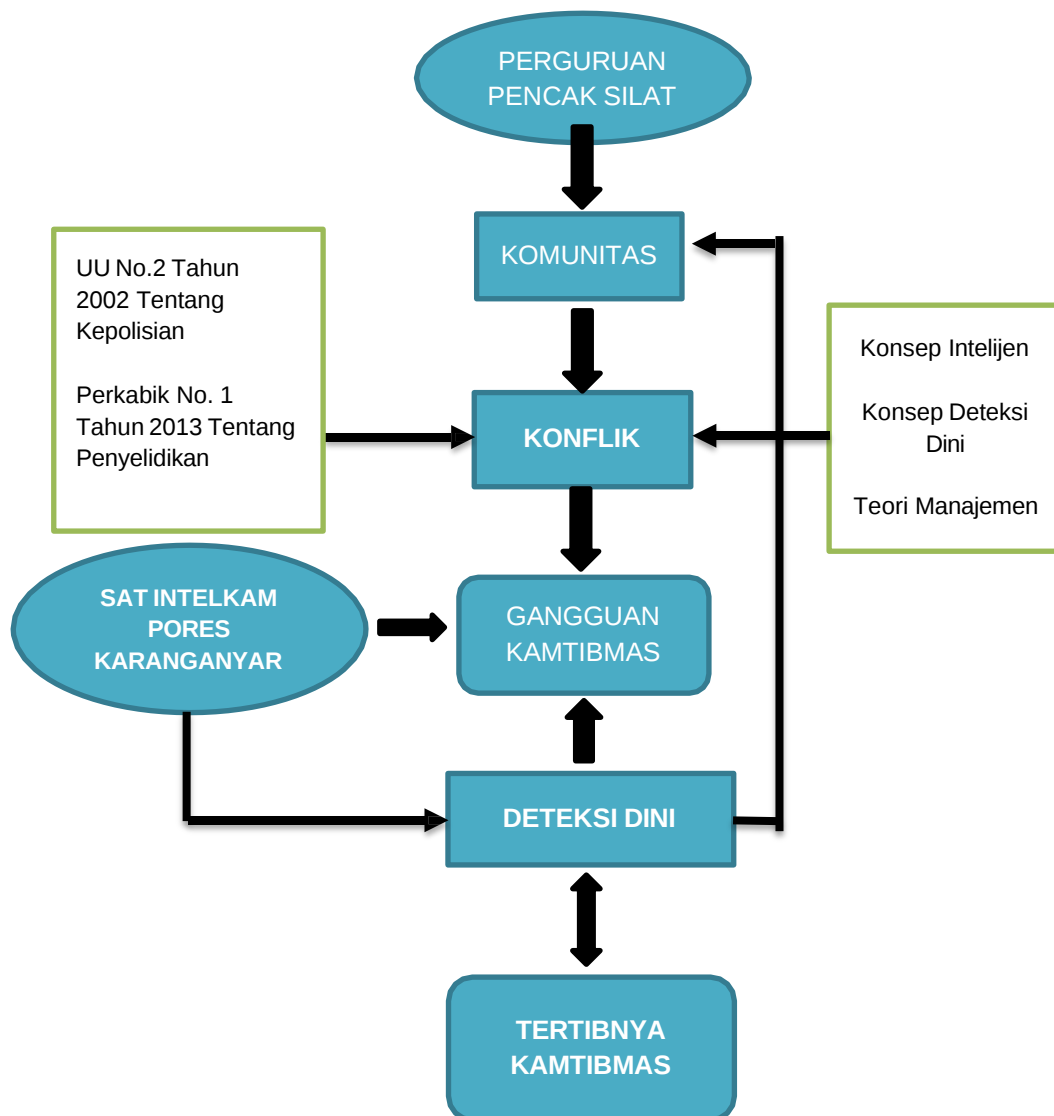
Gambar 2.1 Kerangka Berpikir
